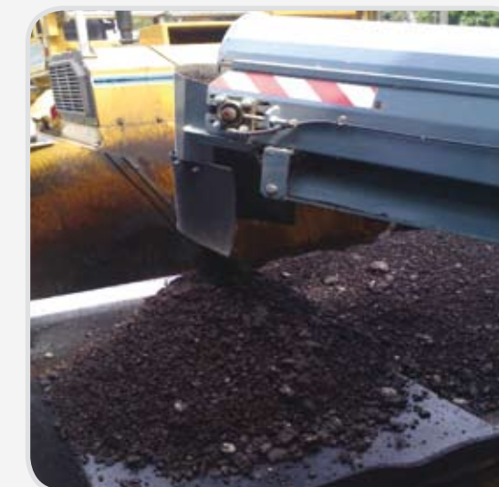
Herstellung von kalt regeneriertem Material
